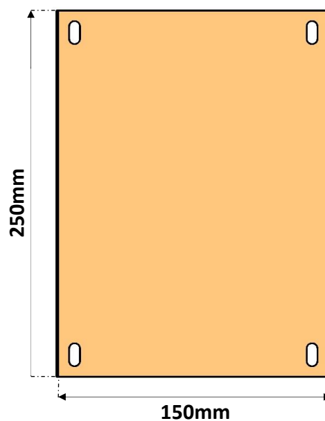
PLACA DE MONTAGEM CHAPA 22# 0,75mm
