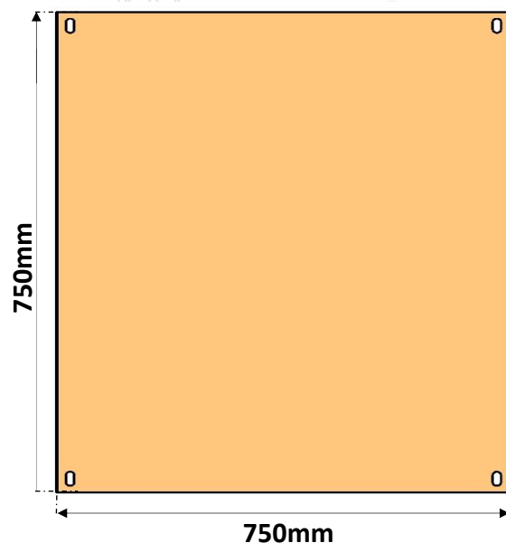
PLACA DE MONTAGEM CHAPA 22# 0,75mm
