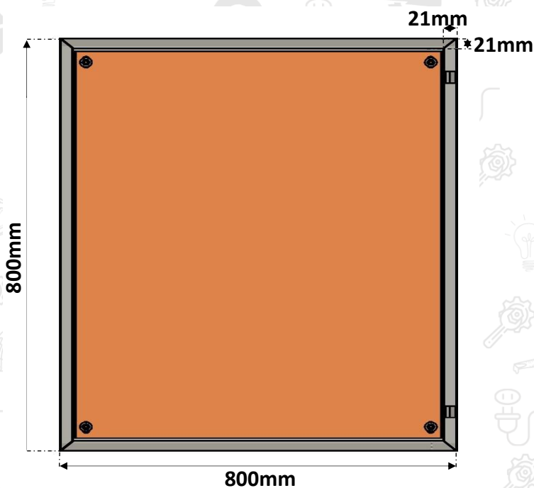
CORPO CAIXA DE MONTAGEM CHAPA 22# 0,75mm
