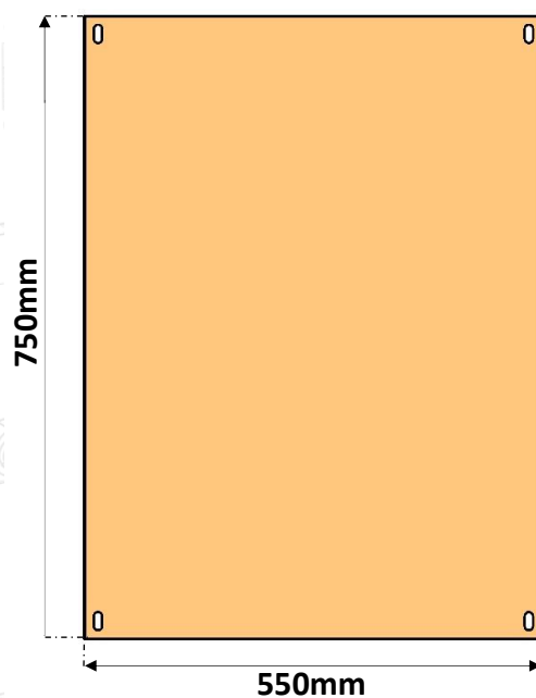
PLACA DE MONTAGEM CHAPA 22# 0,75mm
