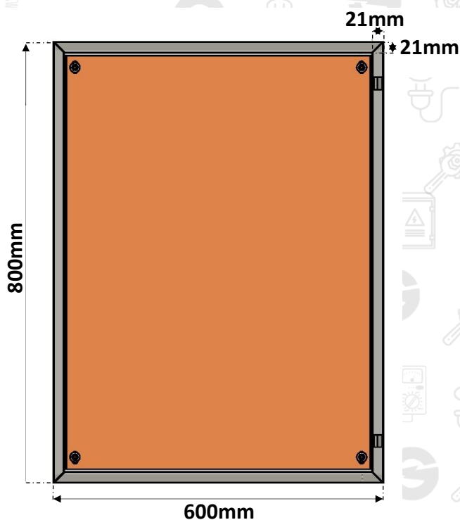
CORPO CAIXA DE MONTAGEM CHAPA 24# 0,60mm
