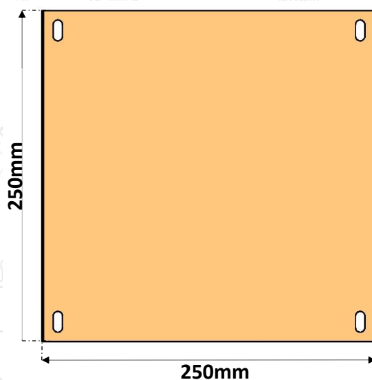
PLACA DE MONTAGEM CHAPA 22# 0,75mm
