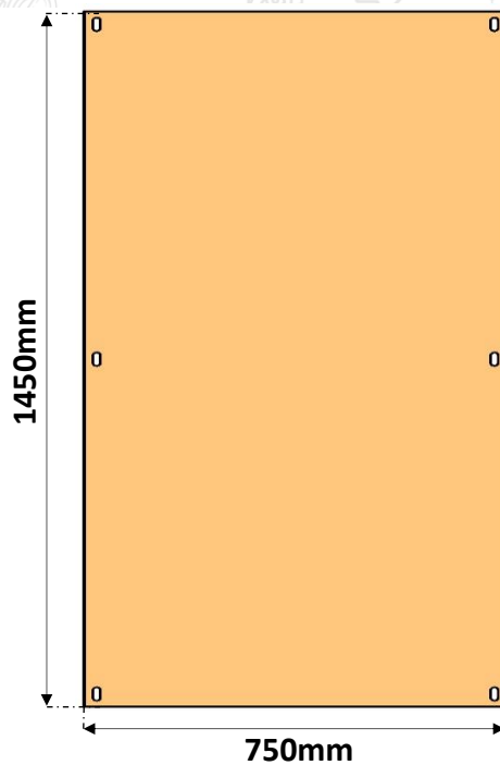
PLACA DE MONTAGEM CHAPA 18# 1,20mm
