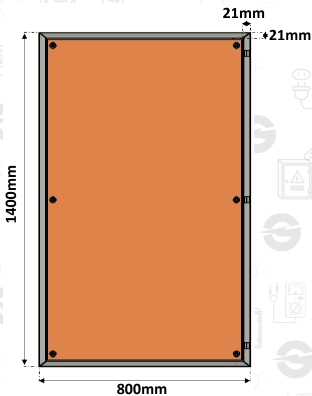
CORPO CAIXA DE MONTAGEM CHAPA 18# 1,20mm
