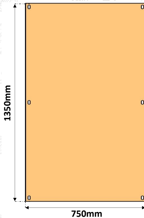
PLACA DE MONTAGEM CHAPA 18# 1,20mm
