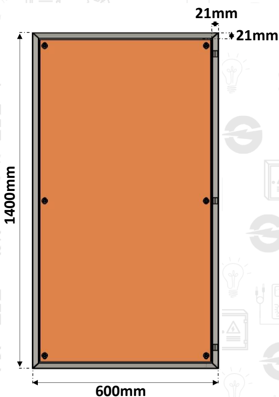
CORPO CAIXA DE MONTAGEM CHAPA 18# 1,20mm
