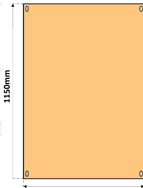
750mm PLACA DE MONTAGEM CHAPA 20# 0,90mm
