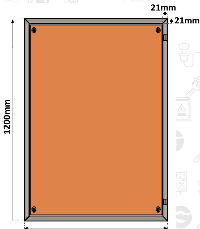
1200mm 800mm CORPO CAIXA DE MONTAGEM CHAPA 20# 0,90mm
