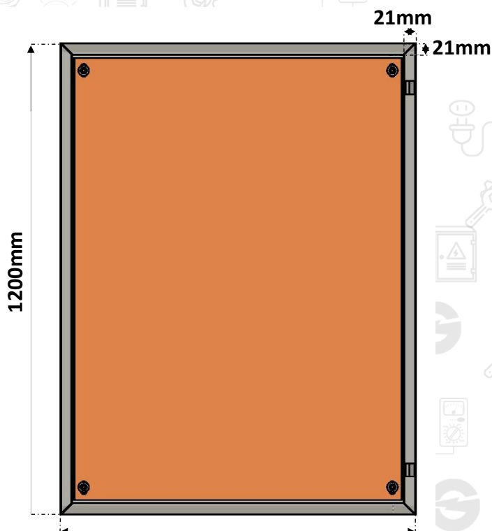
800mm 1200mm CORPO CAIXA DE MONTAGEM CHAPA 18# 1,20mm
