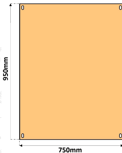
PLACA DE MONTAGEM CHAPA 20# 0,90mm
