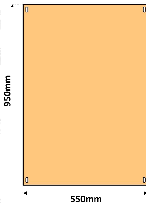
PLACA DE MONTAGEM CHAPA 20# 0,90mm
